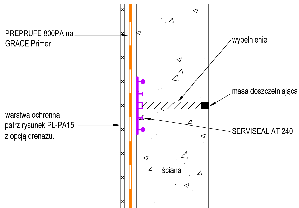
DYLATAcja KONSTRUKCYJNA ŚCIANY
