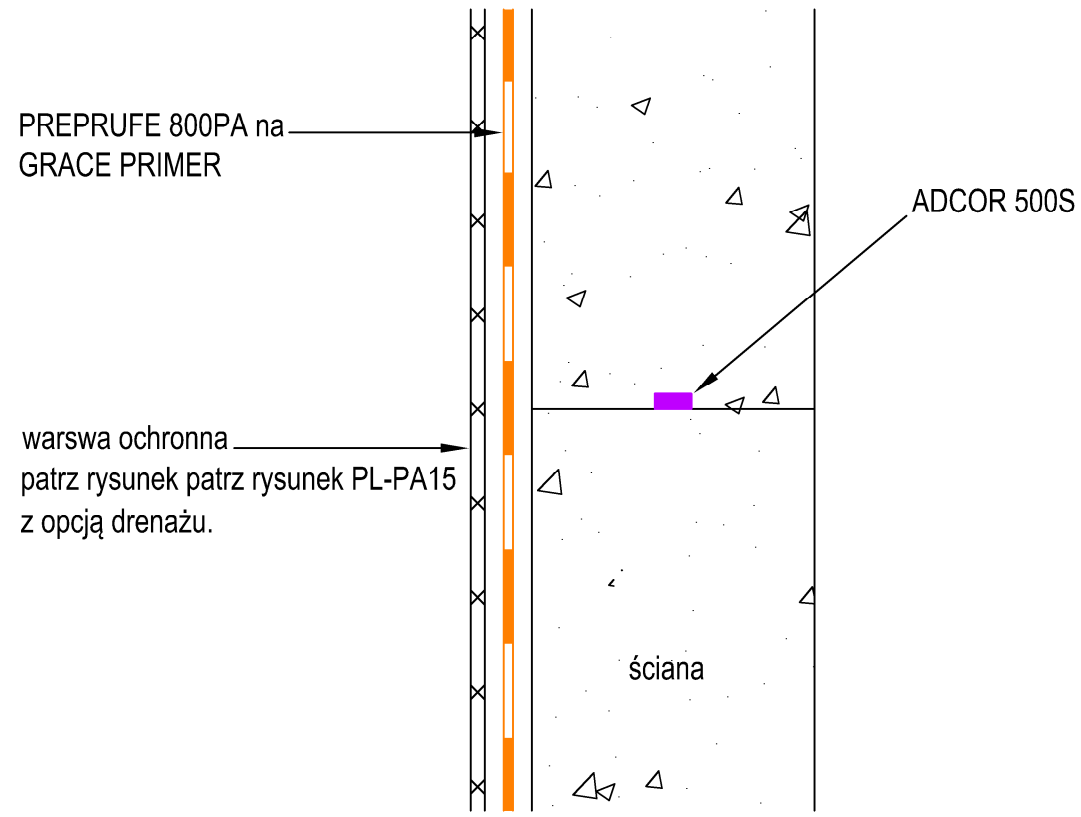
PRZERWA TECHNOLOGICZNA ŚCIANY
